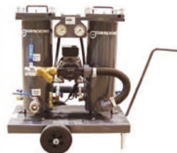
Equipos de Filtraje
